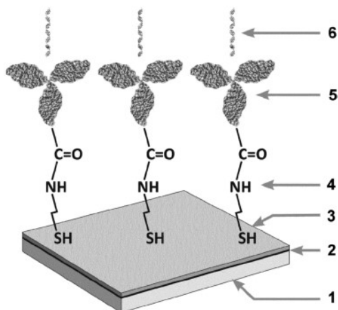
Rys. 1. Schemat budowy biosensora.
