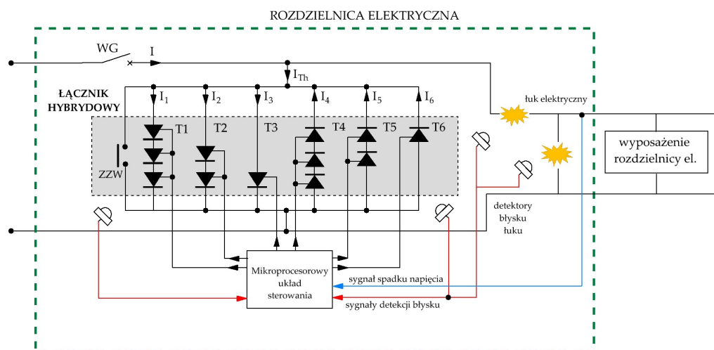
Rys.3. Schemat ideowy eliminatora łuku zbudowany w oparciu o układ zwiernika hybrydowego.
