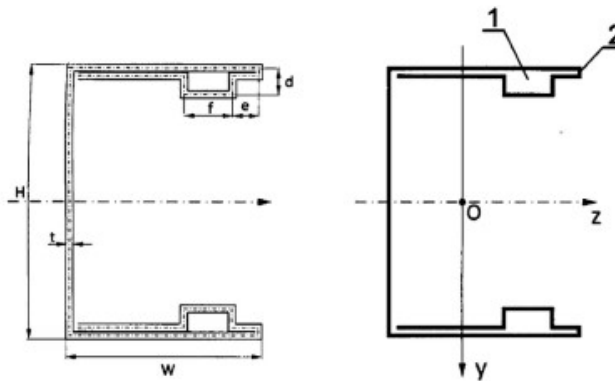
Rys. 6. Cienkościenna belka o przekroju ceowym z prostym środkiem (W.129860).
